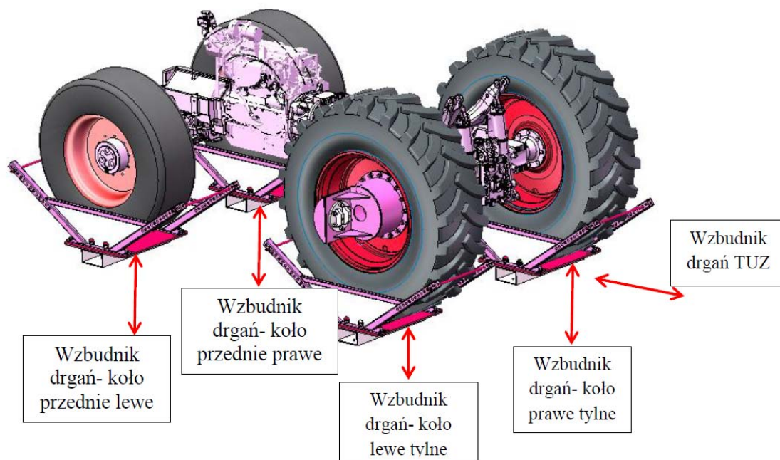
Rys. 1. Mocowanie ciągnika na stanowisku badań
